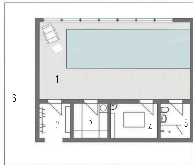
План здания 8x11 м
